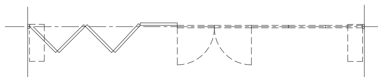
Sidehængt - tofløjet
