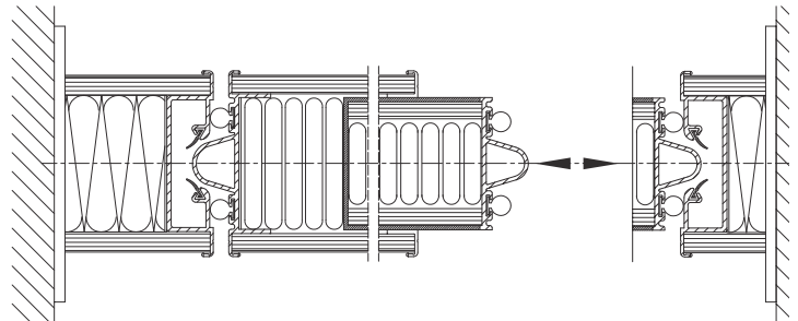
Vægtilslutning
