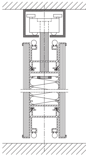
Loft-/gulvtilslutning
