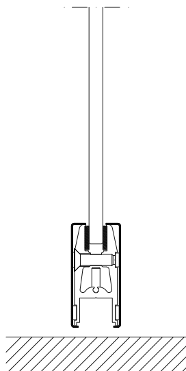
Gulvtilslutning
