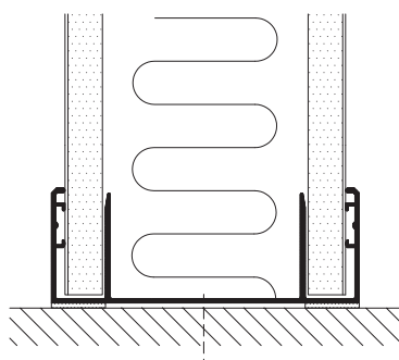
Gulvtilslutning
