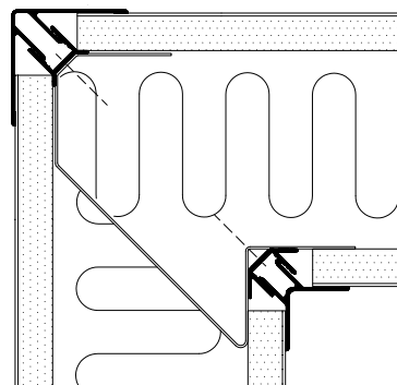
90° hjørne
