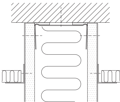
Nedhængt lofttilslutning
