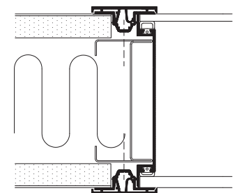
Gipssamling PF 1290
