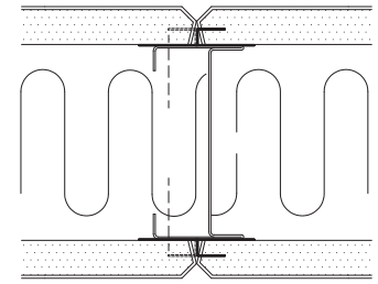
Gipssamling PF 1090
