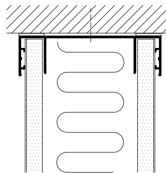
Fast lofttilslutning
