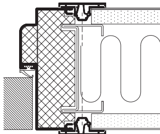
Massivdør
