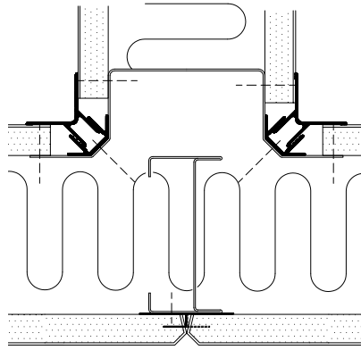
T-samling
